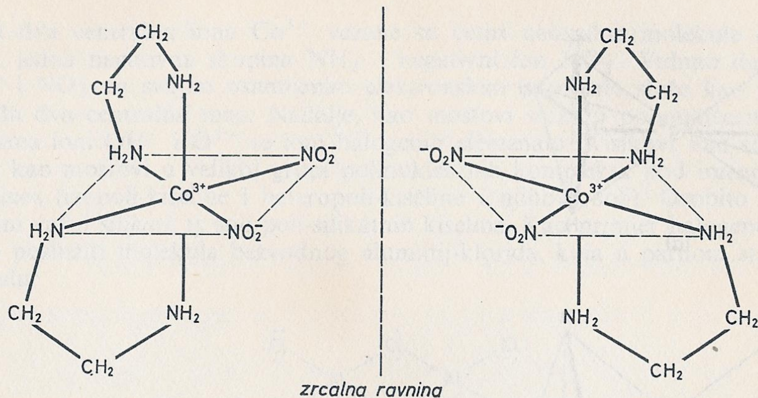
Sl. 6.107. Zrcalna izomerija
